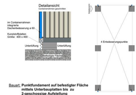
Fundamentschema für Raumcontainer 20'
