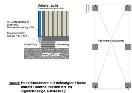
Fundamentalschema für Raumcontainer 20'
